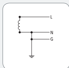
Jednofázová; 3 vodiče
