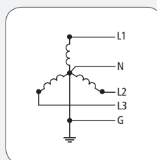
Třífázová; 5 vodičů
