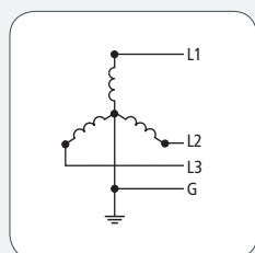
Třífázová; 4 vodiče
