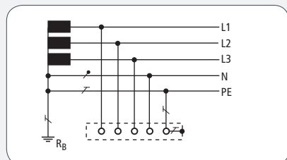
TN-S systém 230/400 V
