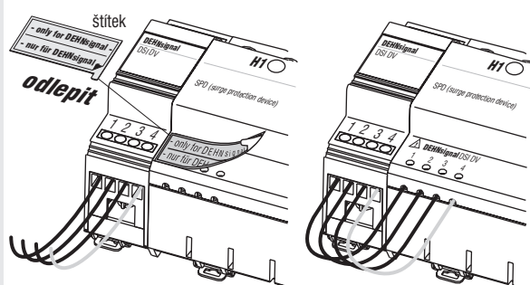
Obr. 5 Připojení
