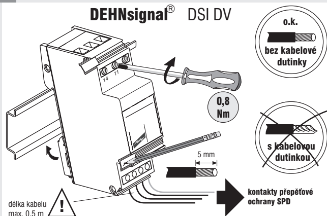
Obr. 5 Připojení
