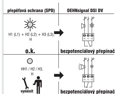
Obr. 3 Signalizace funkčnosti přepětové ochrany
