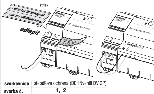
Obr. 6 Instalace DSI DV s přijímacím modulem DSI E DV
