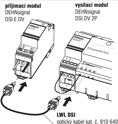
Obr. 6 Instalace DSI DV s přijímacím modulem DSI E DV
