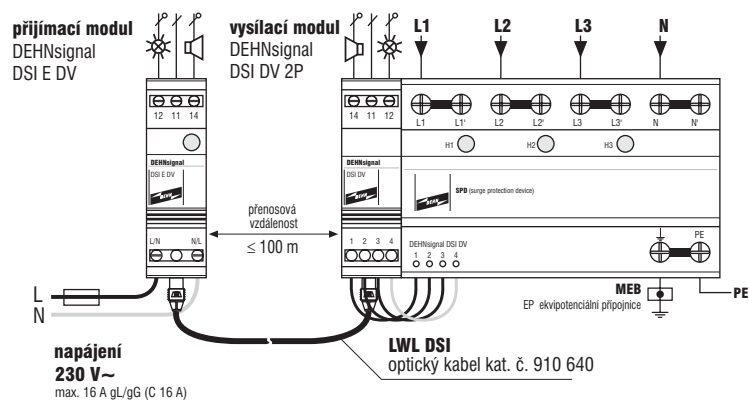
Obr. 6 Instalace DSI DV s přijímacím modulem DSI E DV
