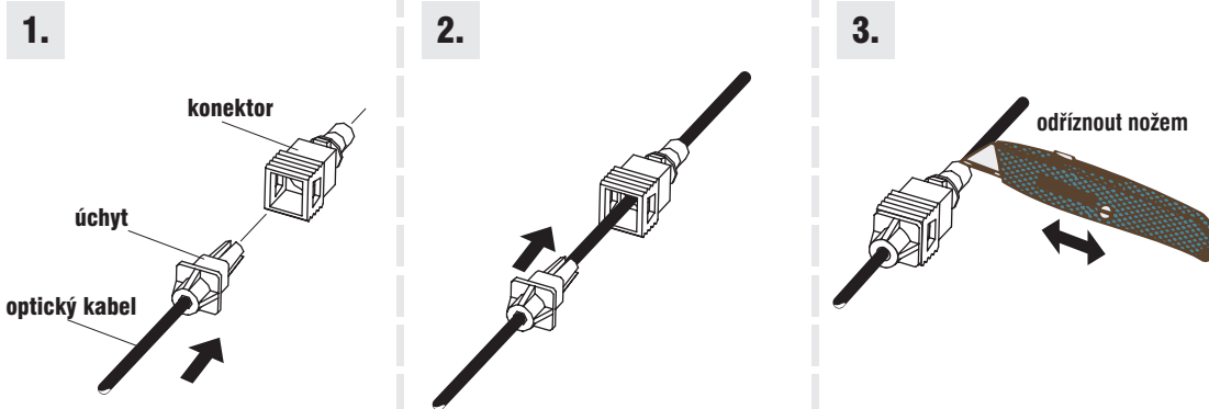
Obr. 6 Instalace DSI DV s přijímacím modulem DSI E DV
