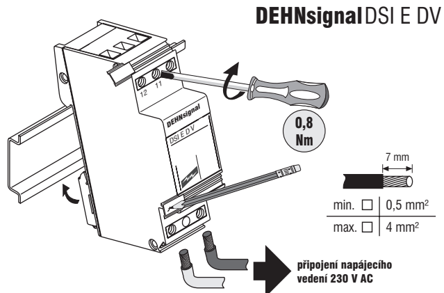
Obr. 2 Montáž a připojení
