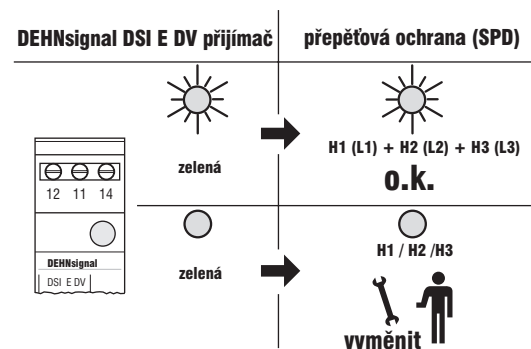
Obr. 7 Signalizace funkčnosti přepětové ochrany
